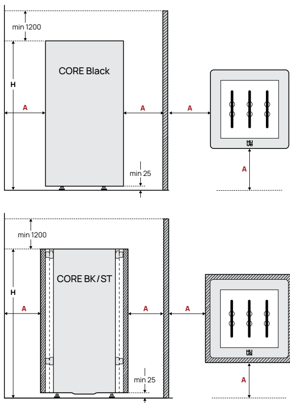
Рисунок 1. Размещение каменки.
