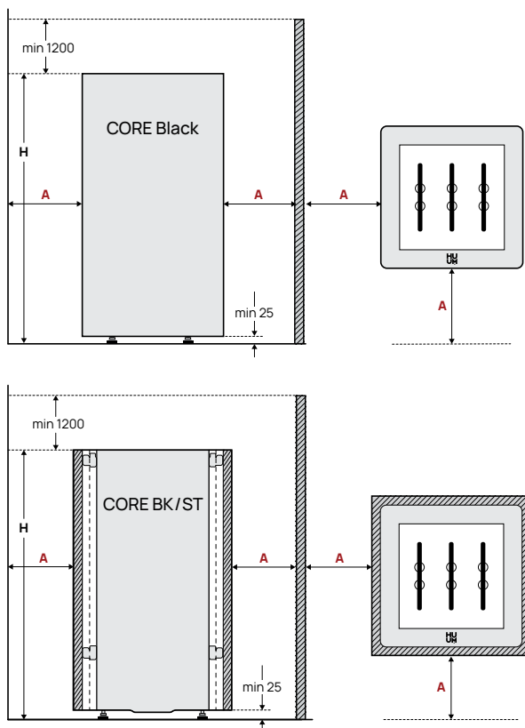
Figur 1. Bastuugnsens placering
