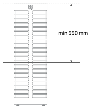
Рисунок 2. Установка каменки HUUM STEEL, частично погруженной в полок.
