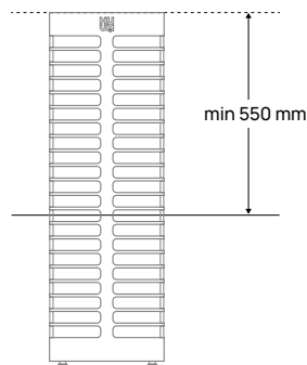
Figur 2. HUUM STEEL bastuugnens montering i svettbänken
