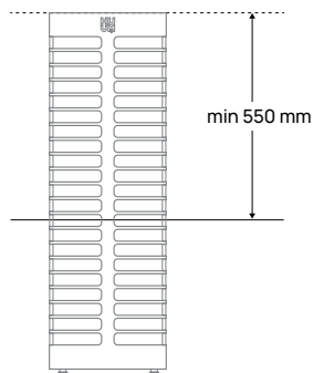
Kuva 2. HUUM STEEL sähkökiukaan upotus lauteisiin
