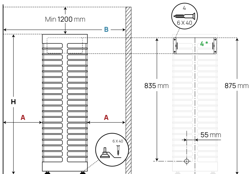
Figur 1 Bastuugns placering
