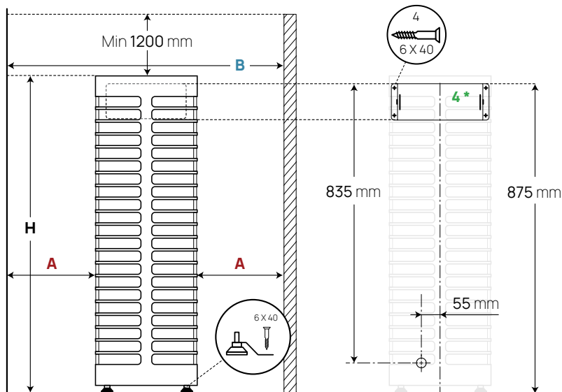
Kuva 1 Kiukaan paikka
