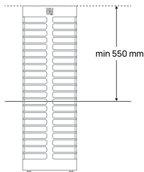
Figure 2. Montage du poêle électrique HUUM STEEL enfoncé dans le banc de sauna
